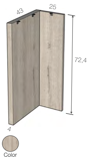
Pm5 Pata madera "L"
