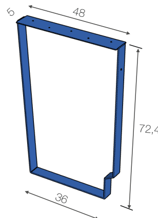
Pm6 Pata metálica
